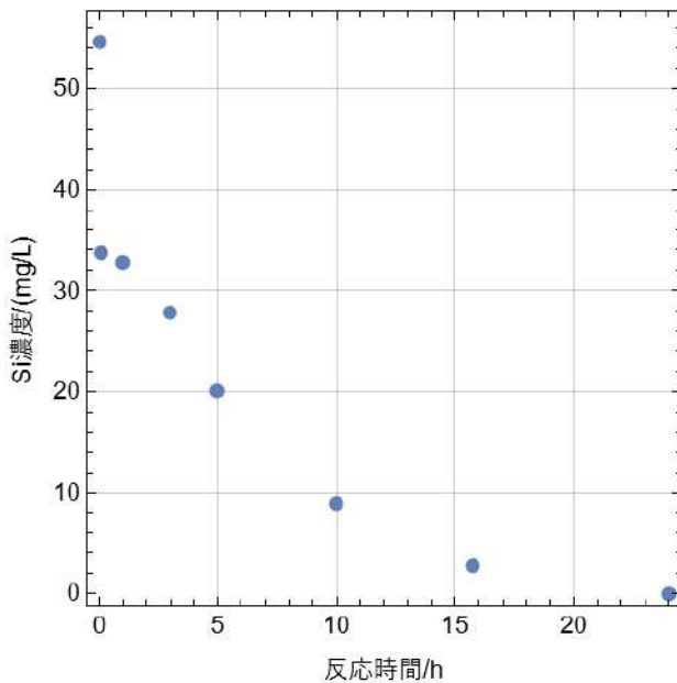
図 10. 酸化マグネシウムによるケイ酸吸着。
