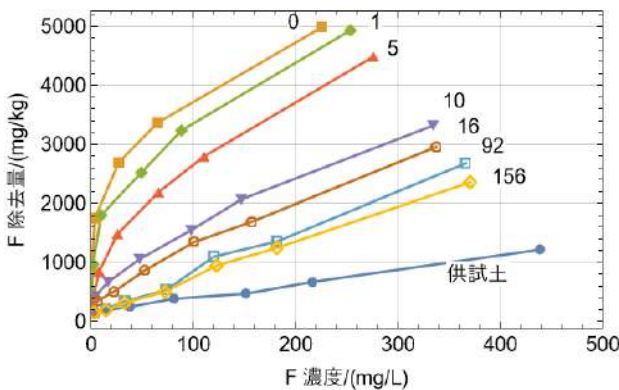
図4. 混合物および供試土のフッ素除去能。
