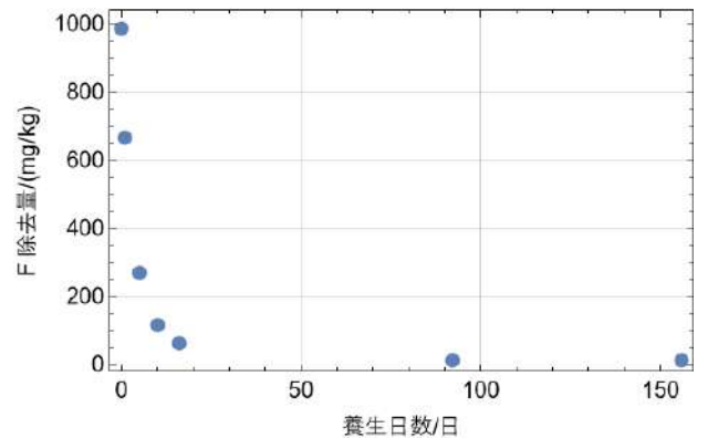
図5. 平衡フッ素濃度 0.8 mg/L におけるフッ素除去量。
