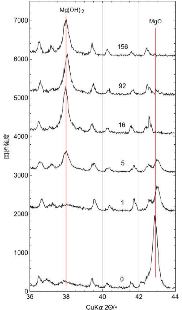
図 7. <105 μm 画分の粉末 X 線回折図形。
