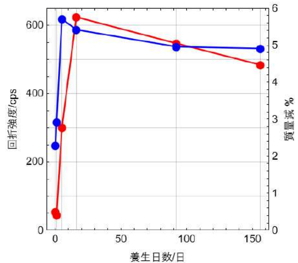
図9. 2\theta = 38^\circ におけるピークの強度(赤丸)と 300^\circ\text{C} \sim 400^\circ\text{C} における減量率(%) (青丸)の養生日数に伴う変化。
