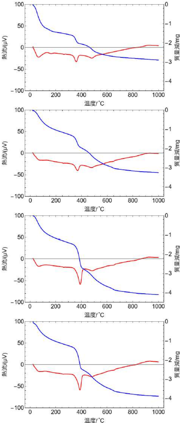
図8. 上から0日、1日、5日、16日後の熱分析結果。
