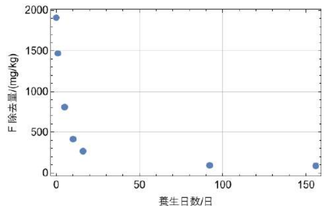
図6. 平衡フッ素濃度 8 mg/L におけるフッ素除去量。
